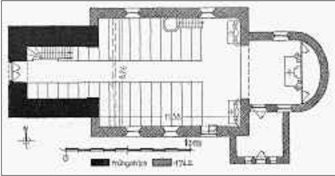
Kath. Pfarrkirche. Grundriss
